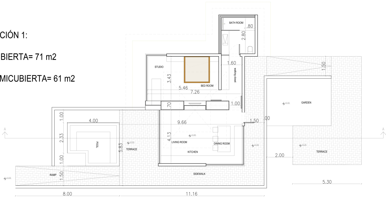
PLANTA ARQUITECTONICA
