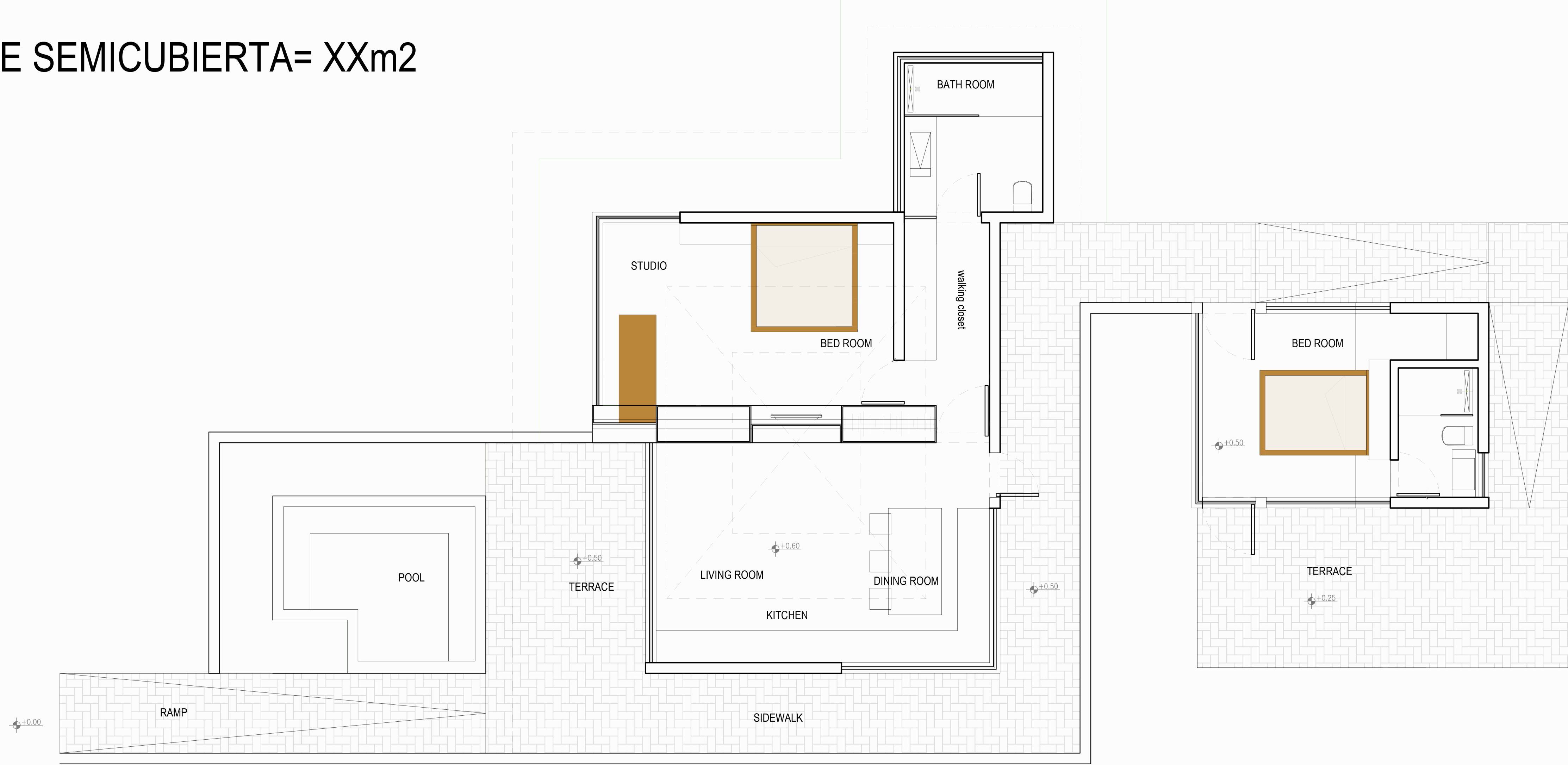
PLANTA ARQUITECTONICA
