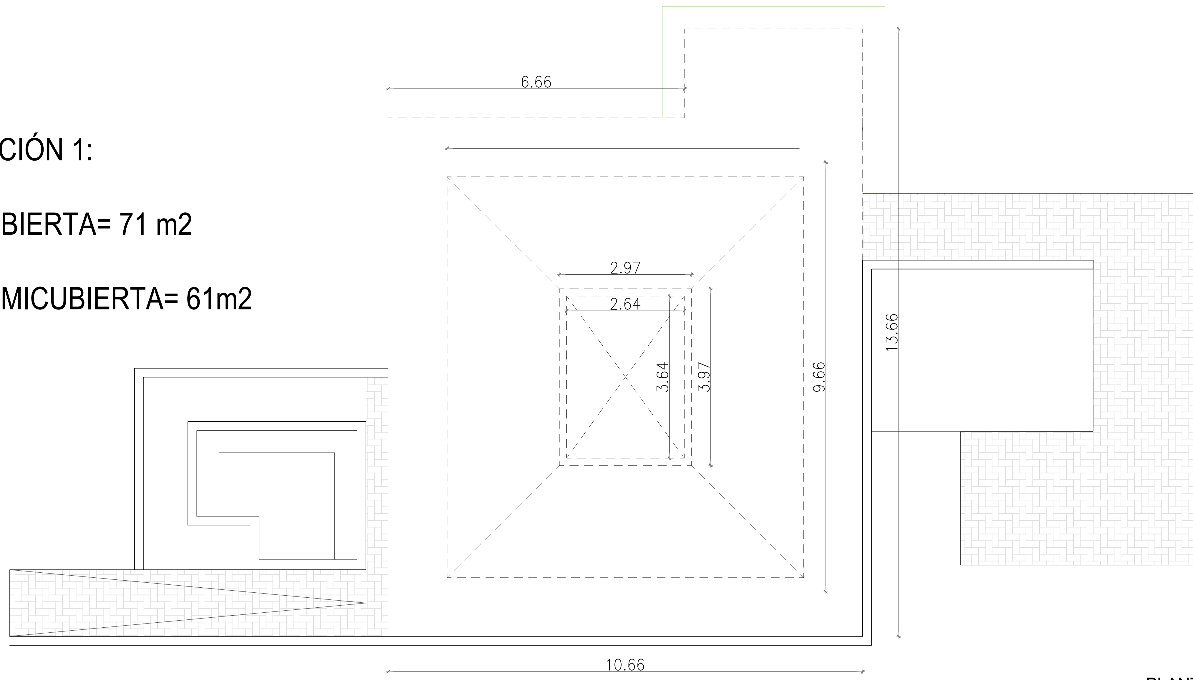
PLANTA TECHOS
